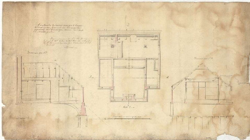
Bouwtekening uit ca. 1860 voor het tolhuis van Mensingeweer (BbG).
